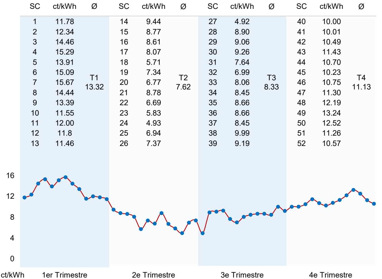
Évolution du prix du marché suisse de l'électricité en 2025
